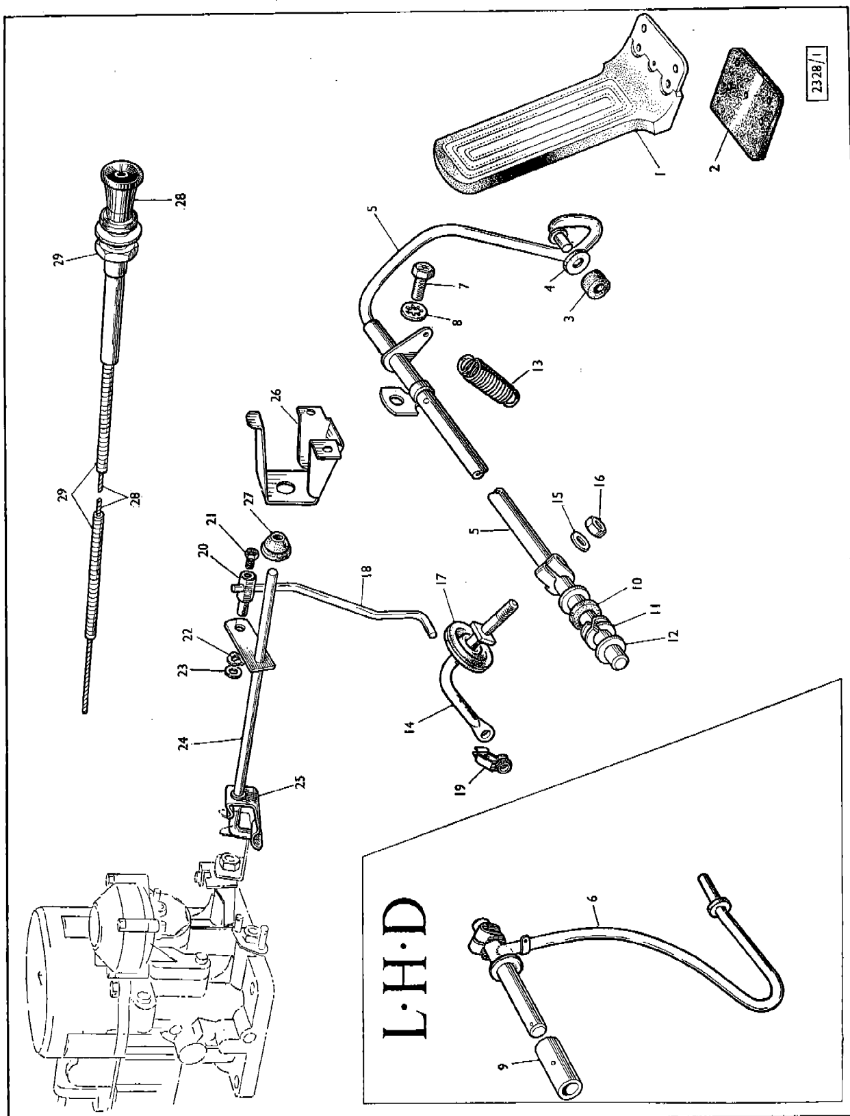
SECTION DA
