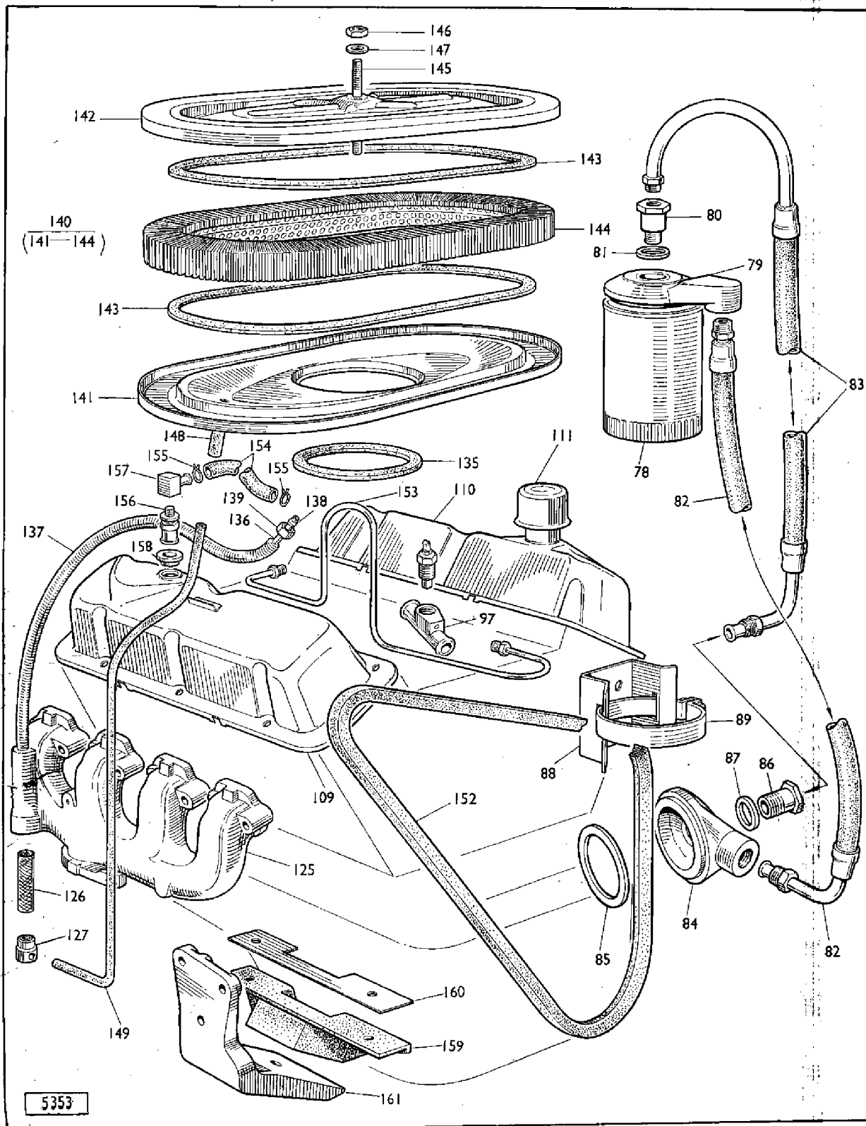
PLATE D — SECTION AF
